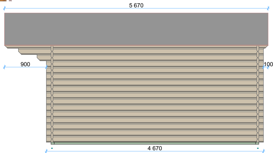
Façade D
